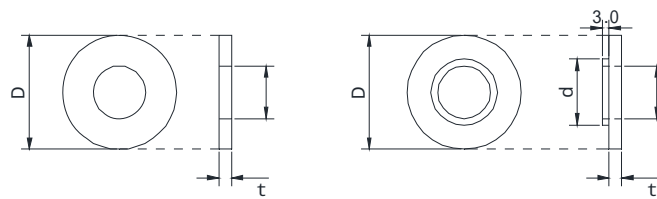
図 - 2.9 アンカープレート止めワッシャー標準図
