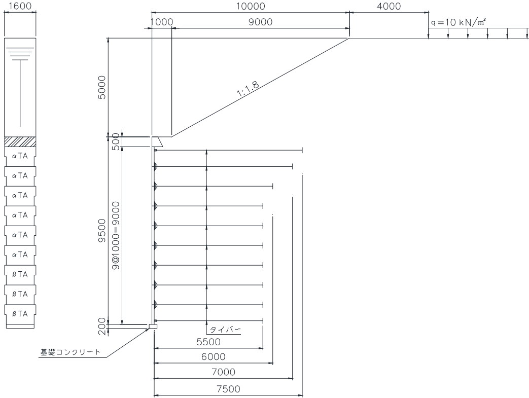
図 3 - 1 計算対象の多数アンカー式補強土壁
