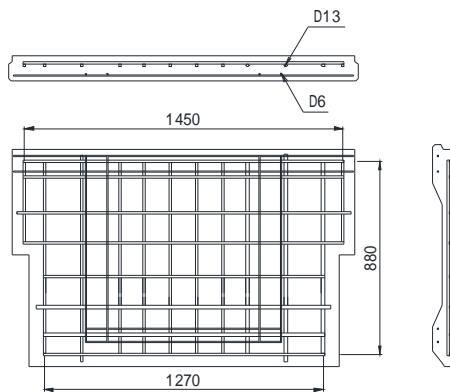
(b) (中層タイプ)
