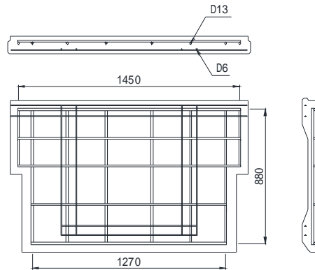
(a) (浅層タイプ)
