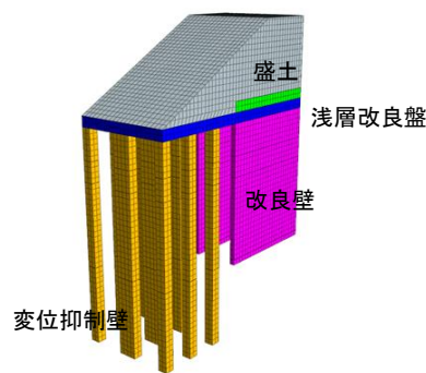
図-2 変位抑制壁付き壁式改良工法
