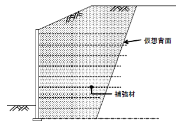
図-6 仮想背面
