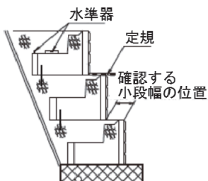
写真-3 最下段の箱体据付 図-8 各段の箱体設置
