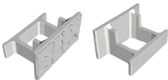
図-2 箱体形状
