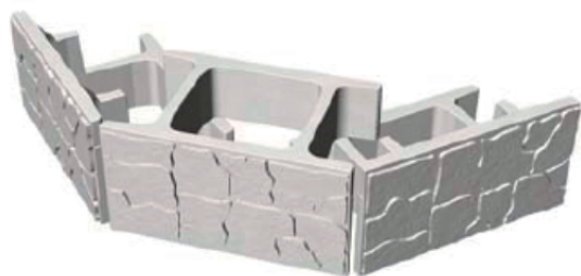
図-3 外曲げ部の設置例
