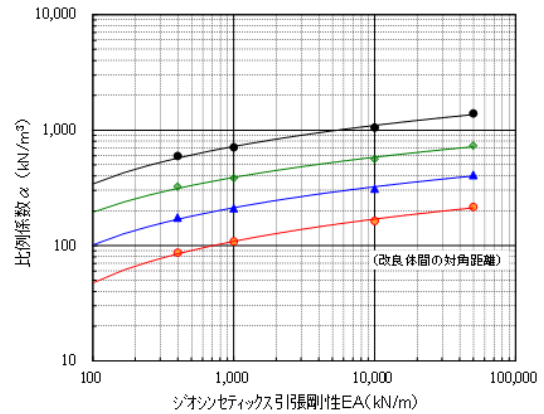
図-6 比例係数αとジオテキスタイルの引張剛性の関係
