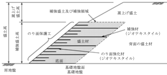
(a) のり面勾配1:1.0より緩い場合
