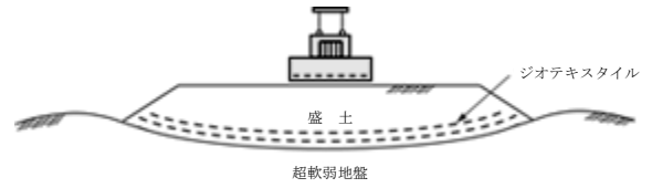
(a) 敷設工法
