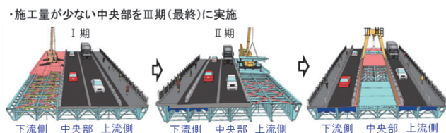
図-4 遅延リスクを低減する施工手順の採用
